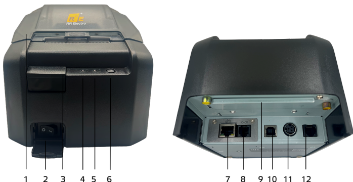
Рисунок 1. Внешний вид ККТ
