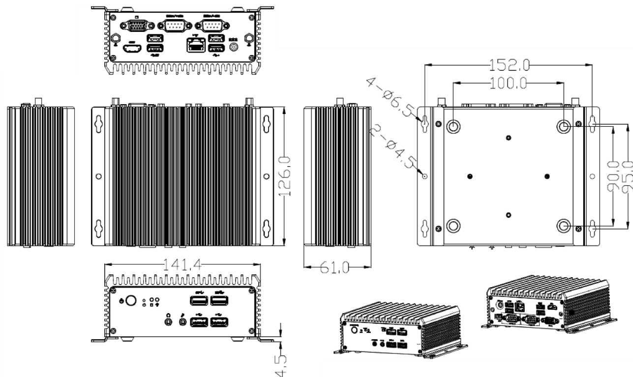
Рисунок 2. Габаритные размеры
